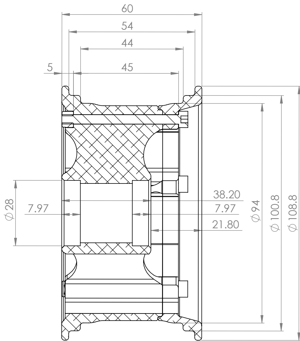
SECTION A-A SCALE 1 : 1
